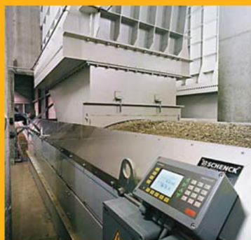
Pesage dynamique de minéraux au Sénégal
